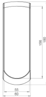
Draufsicht
