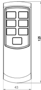
Draufsicht Top view
