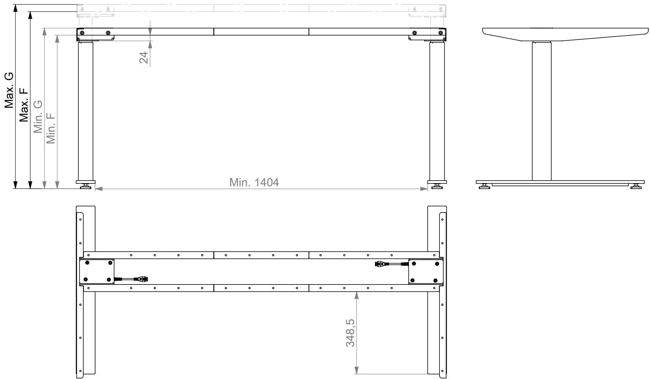
Fixer Tischrahmen in L - Form mit Fußtyp B Desk frame fix in L - Shape with foot type B
