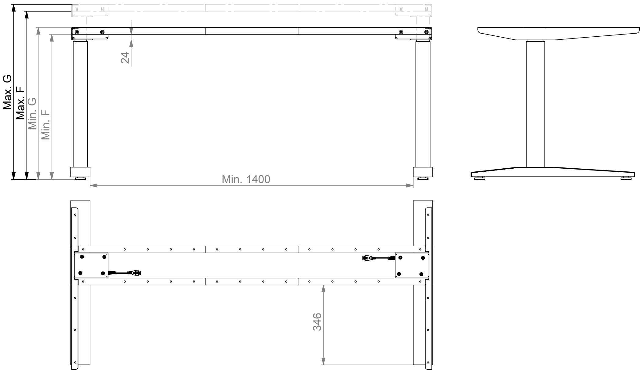
Fixer Tischrahmen in L - Form mit Fußtyp A Desk frame fix in L - Shape with foot type A
